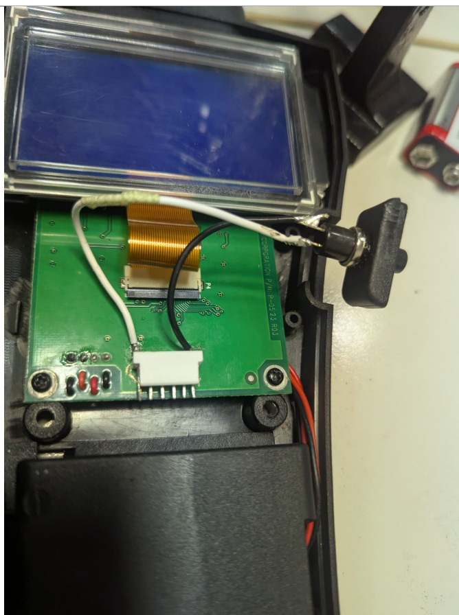
Fig 1 Pulsador de power adaptado al instrumento
