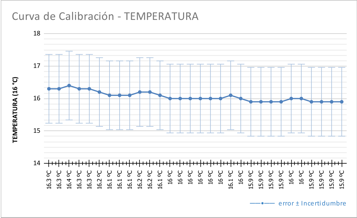
Curva de Calibración 16 °C
