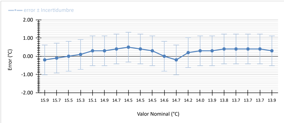
Curva de Calibración 15 °C
