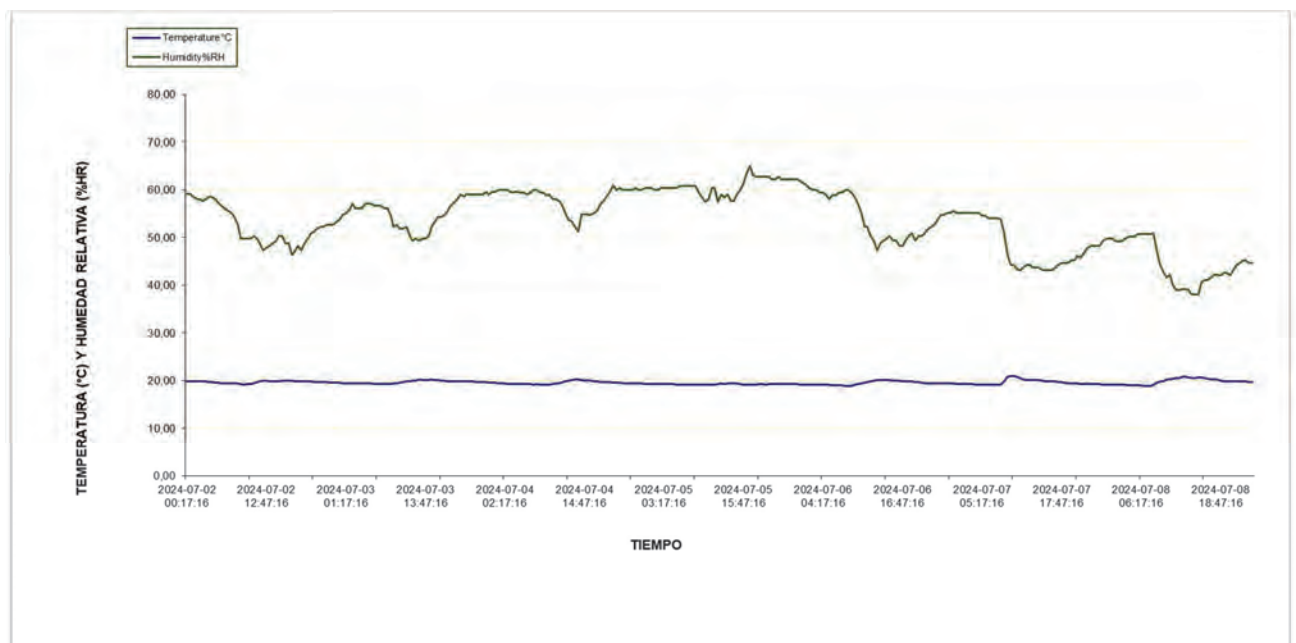
Gráfico 1: Sensor patrón #1
