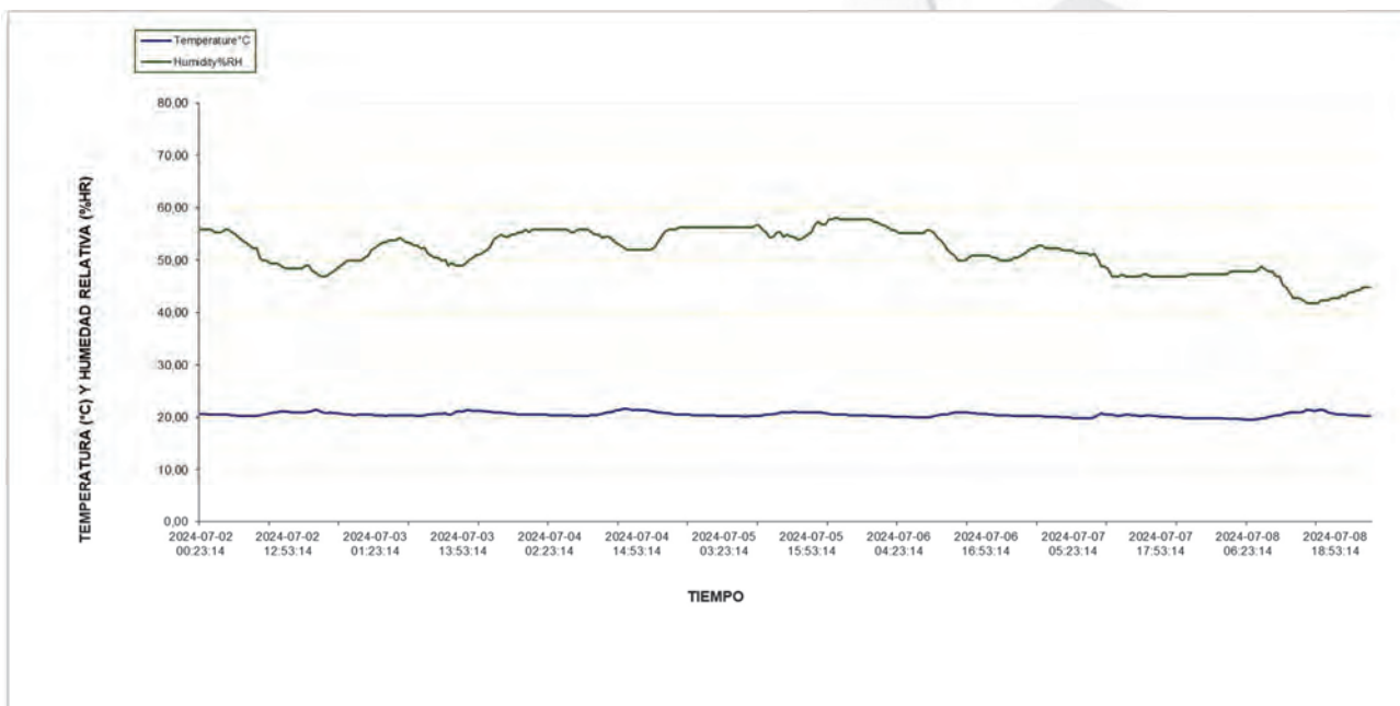
Gráfico 15: Sensor patrón #15
