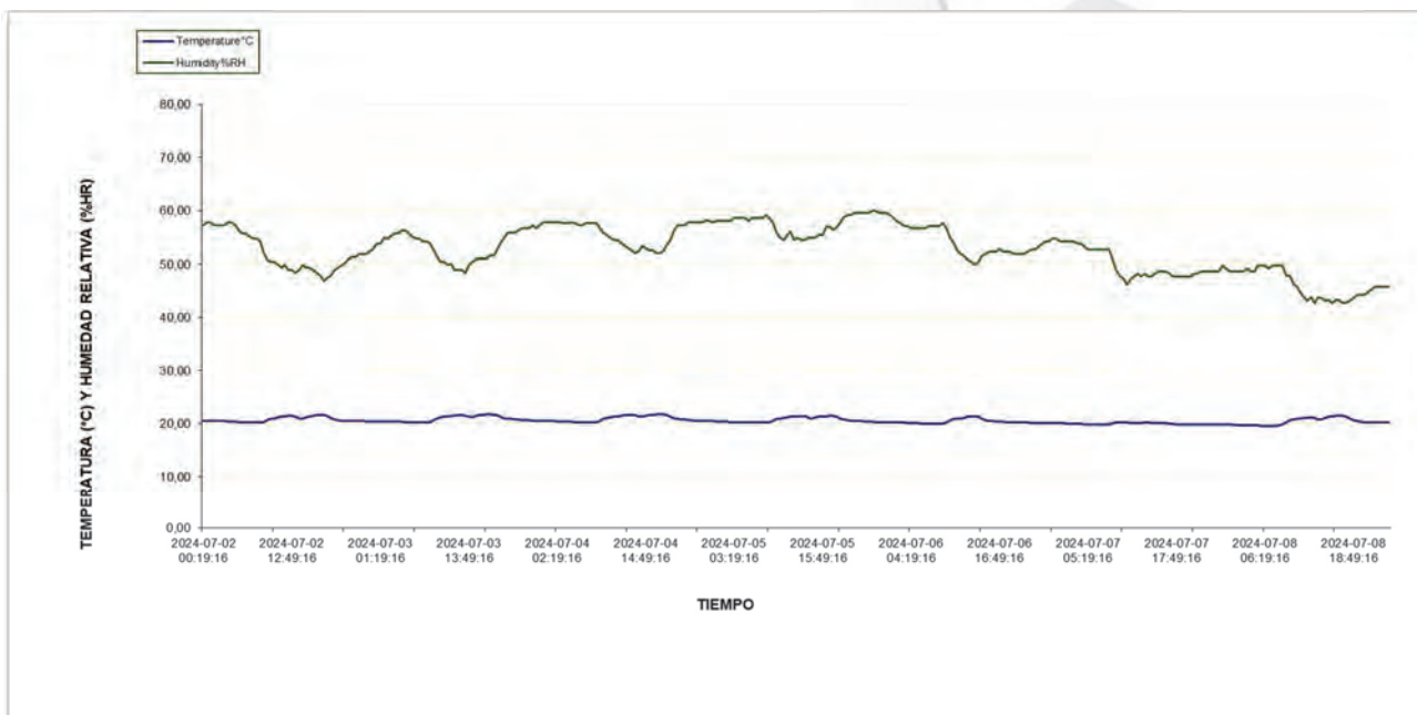
Gráfico 5: Sensor patrón #5
