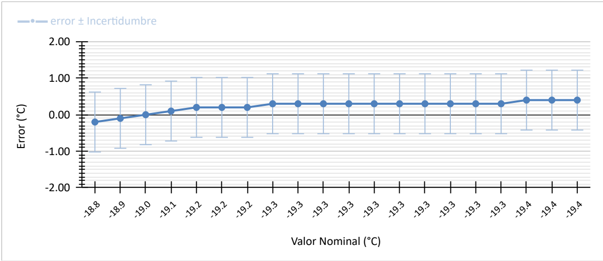
Curva de Calibración -19 °C
