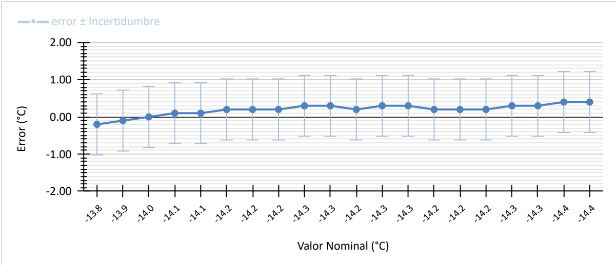
Curva de Calibración -14 °C
