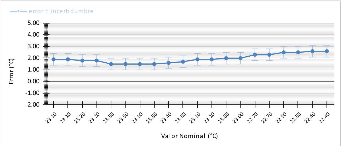
Curva de Calibración 25 °C
