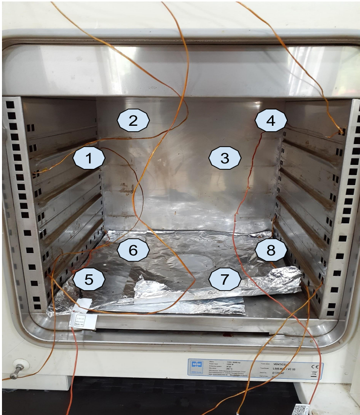
Diagram de Posición de Sensores (Sensor Position Diagram)
