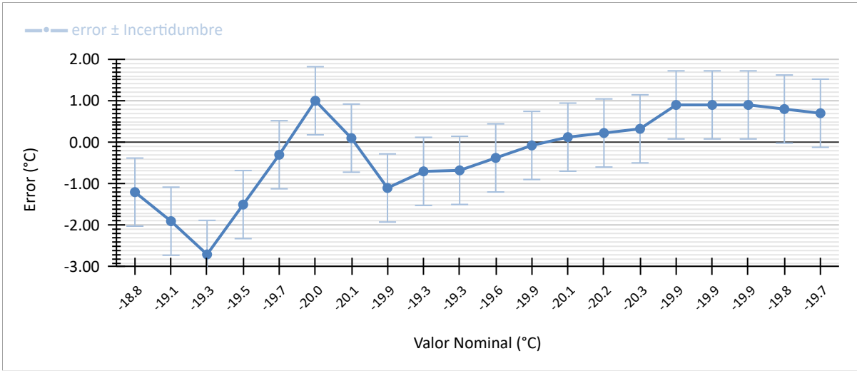
Curva de Calibración -20 °C
