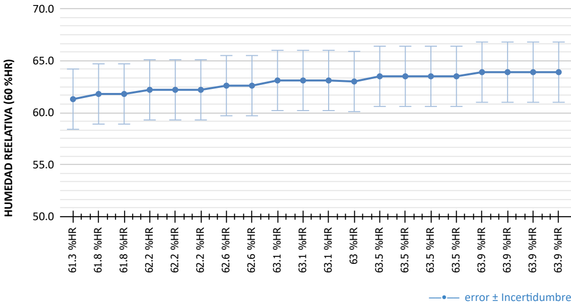
Curva de Calibración - HUMEDAD
