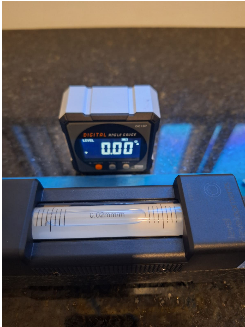
Fig 2 Medición del desplazamiento en segunda posición
