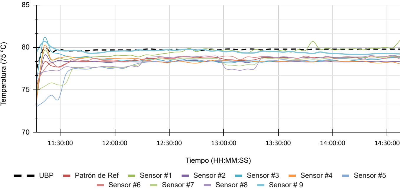
Caracterización de Temperatura en 80 °C - Proc. Cocción, Tiempo: 3h 23 min
