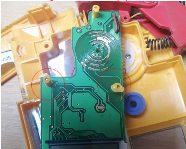
Figura 3: Remaches rotos.
