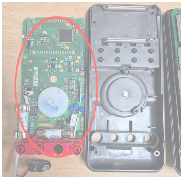
Figura 1. Placa dañada del multímetro.
