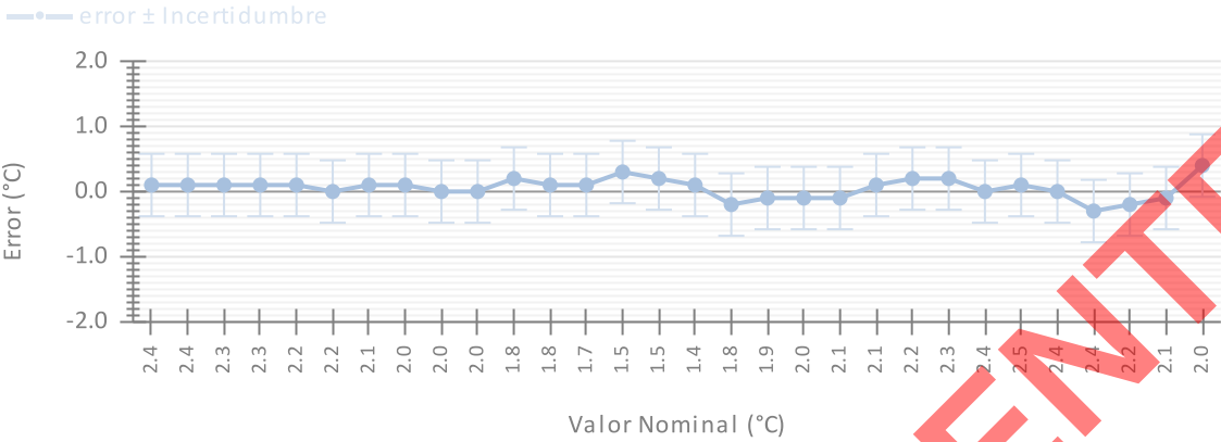
Curva de Calibración - TEMPERATURA 2°C
