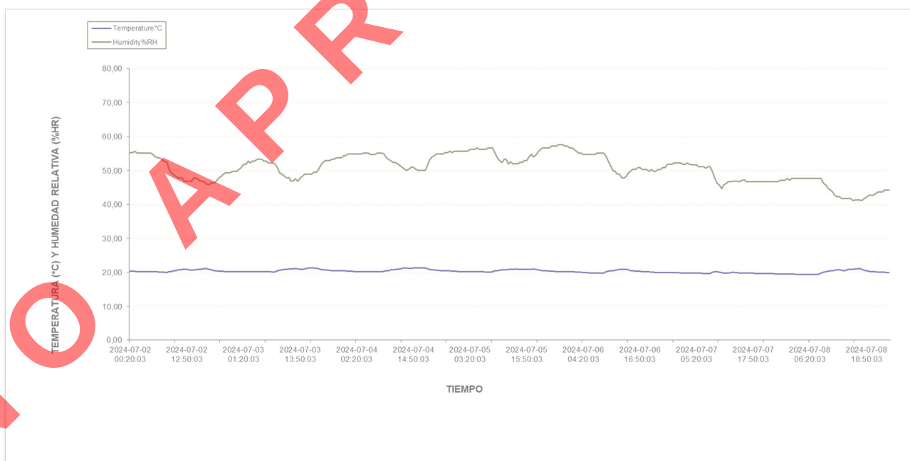
Gráfico 7: Sensor patrón #7
