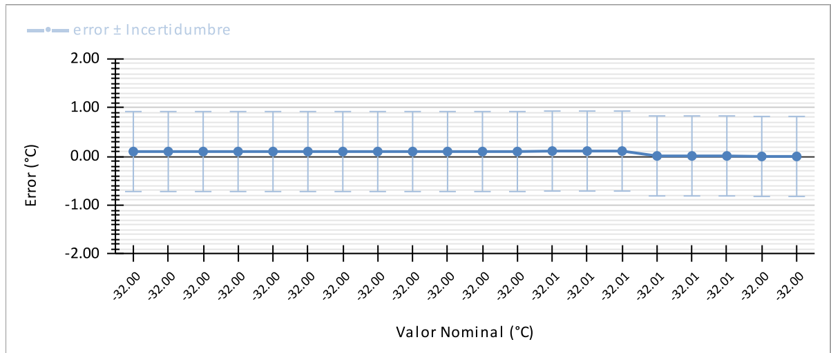
Curva de Calibración -32 °C
