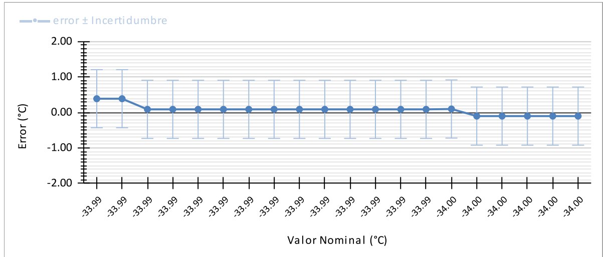
Curva de Calibración -34 °C
