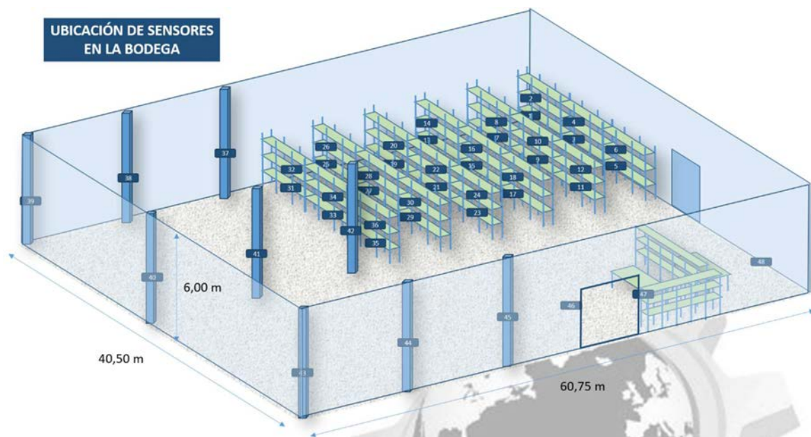
Figura #1: Diagrama de posición de sensores
