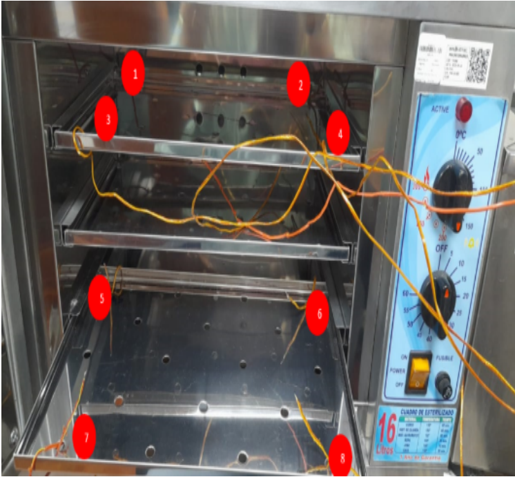
Diagram de Posición de Sensores (Sensor Position Diagram)
