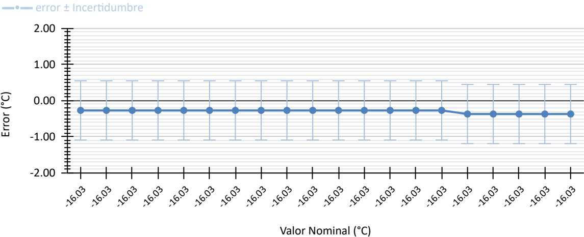
Curva de Calibración -16 °C
