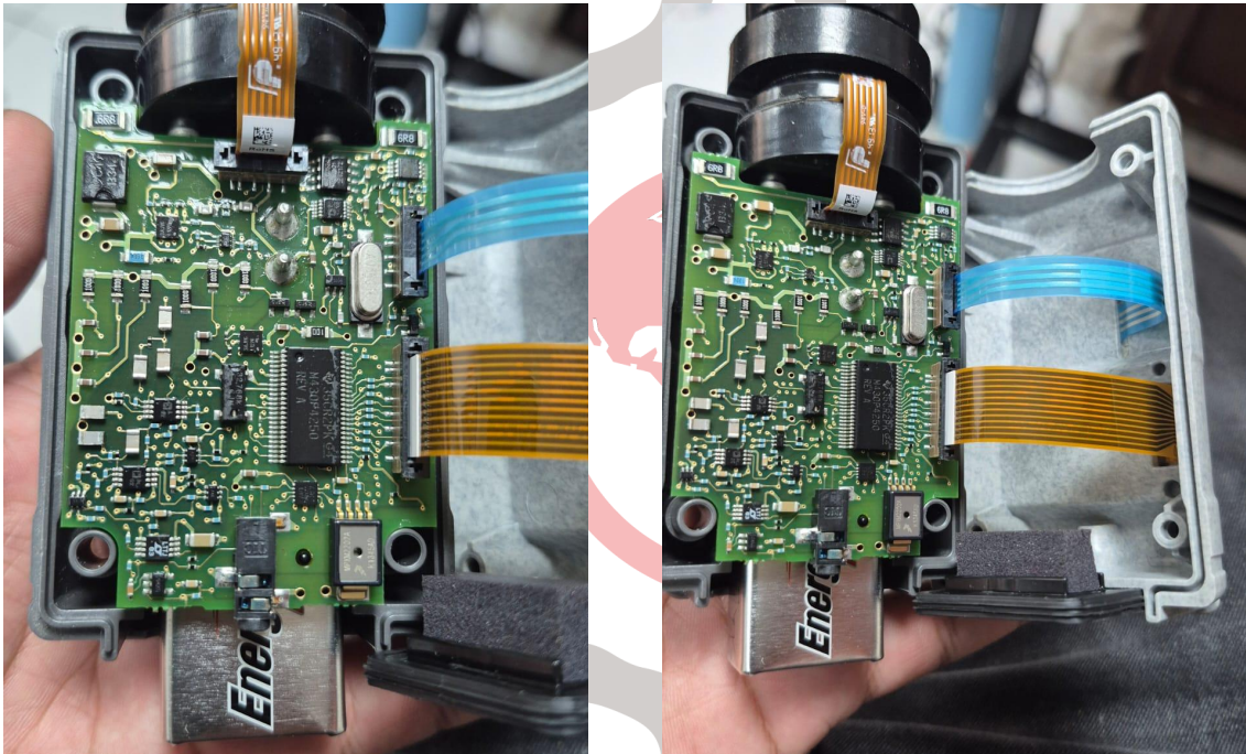
Figura 2. Placa electrónica.
