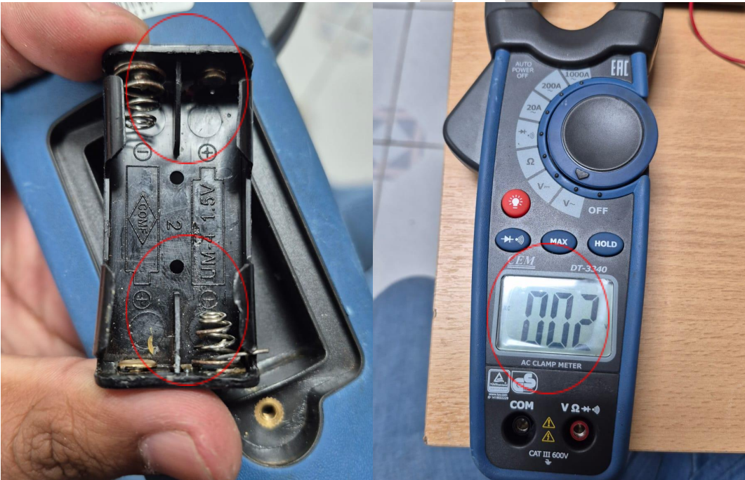
Figura 2. Bornes arreglados y el estado de la placa del dispositivo indicador..
