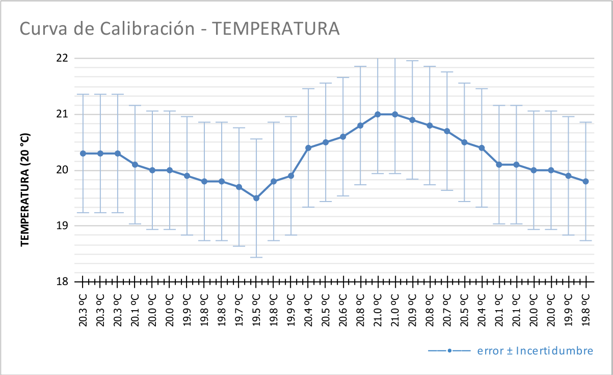
Curva de Calibración 20 °C
