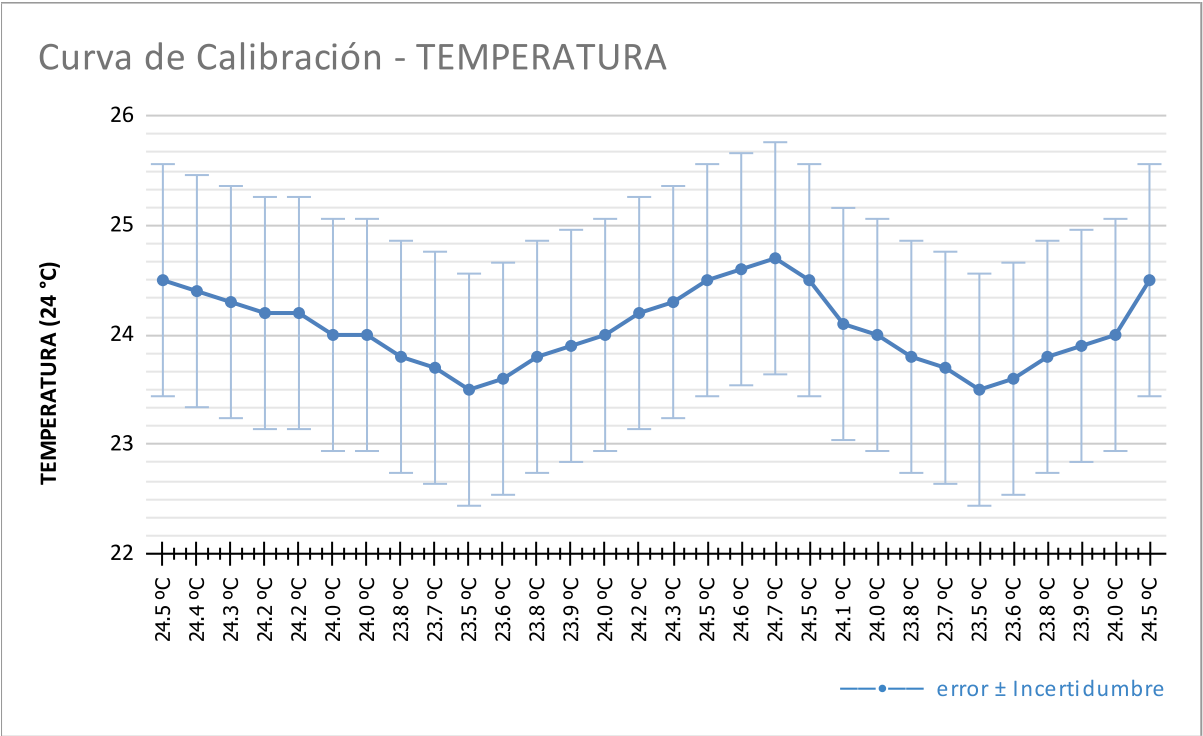
Curva de Calibración 24 °C
