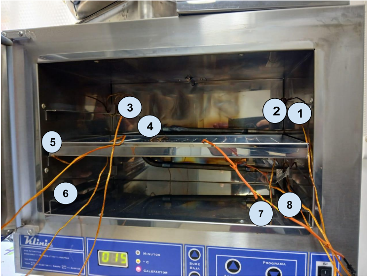
Diagram de Posición de Sensores (Sensor Position Diagram)
