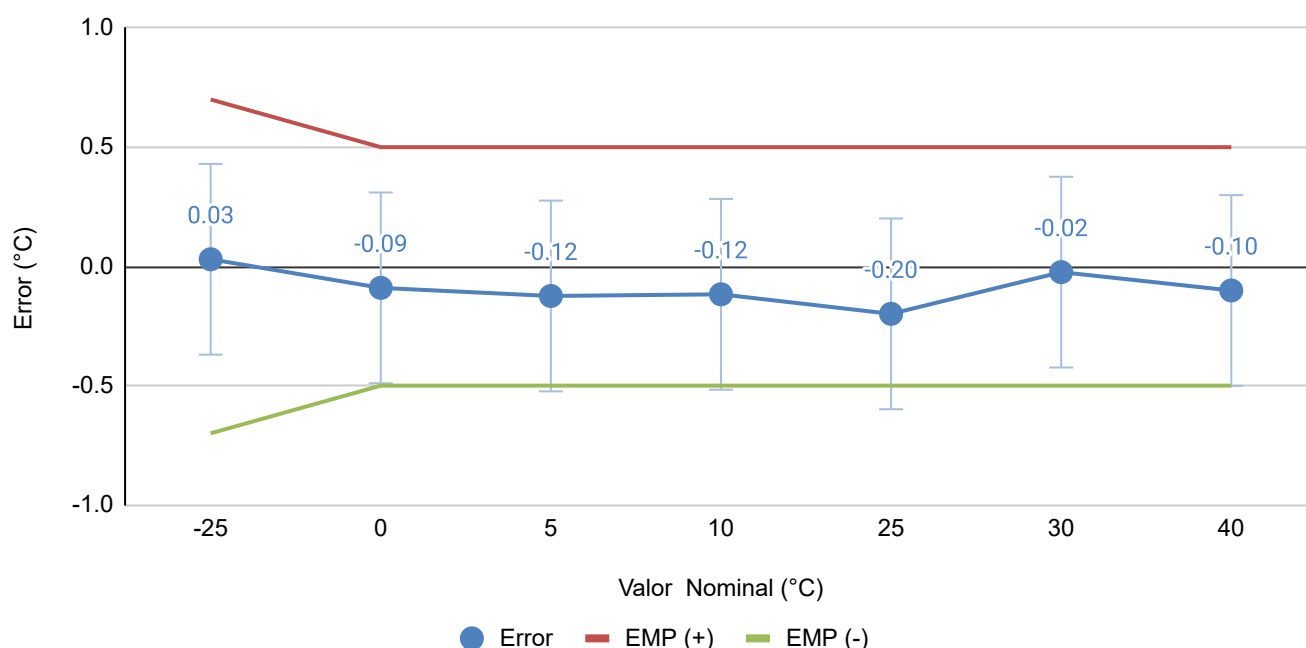
Curva de Calibración
